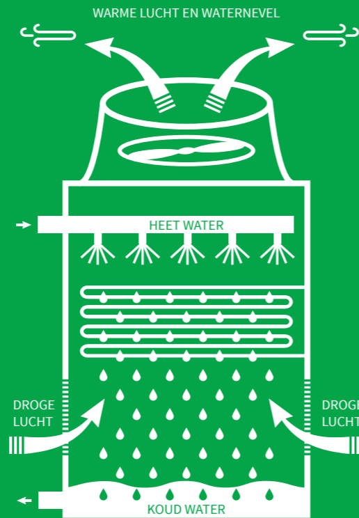
Natte koeltoren
